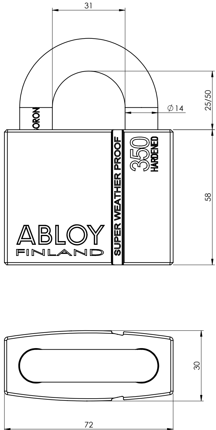
PLI350T
